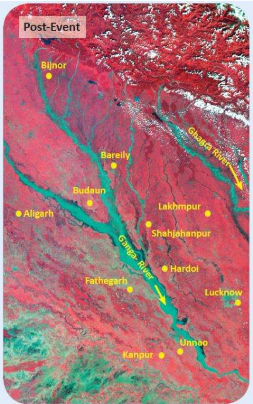
IRS-P6 AWiFS 29 Sep-2010
